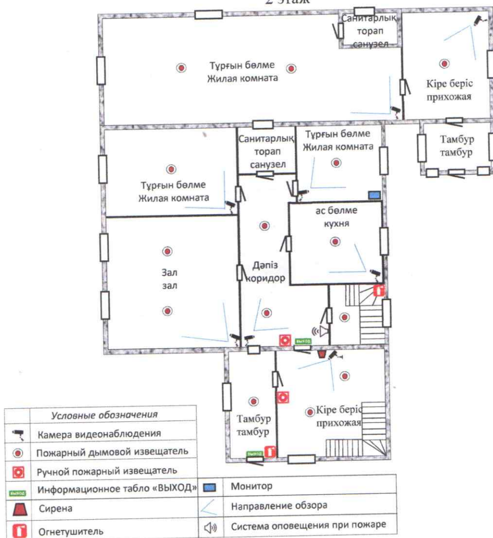
Схема размещения видеонаблюдения, тревожной кнопки, системы оповещения 2 этаж
