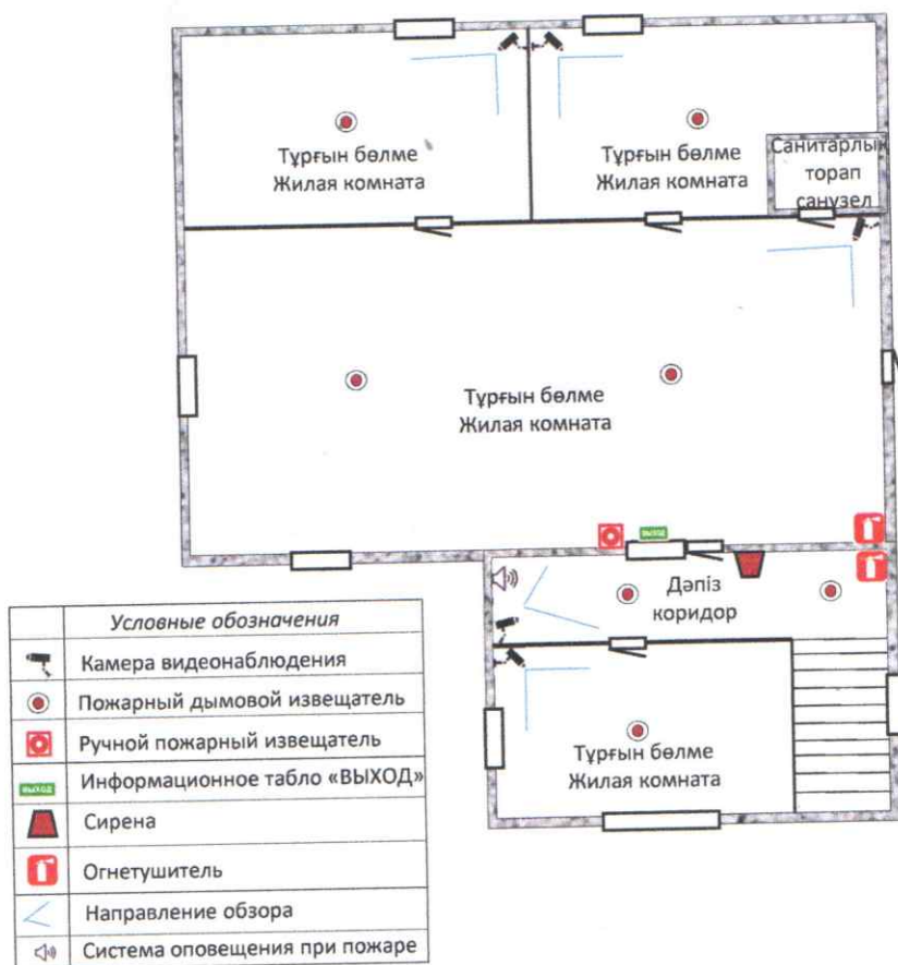
Схема размещения видеонаблюдения, тревожной кнопки, системы оповещения 3 этаж
